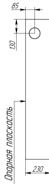
Вид слева
